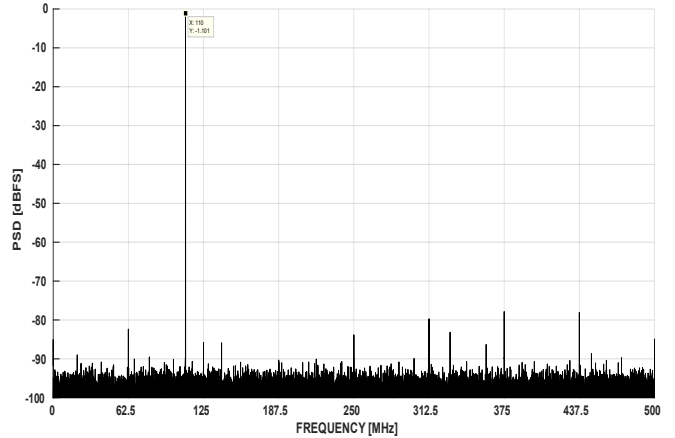
图 7-16. FFT at Fin = 110MHz, 1GSPS (1Vpp FS)
