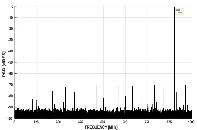
图 7-14. FFT at Fin = 900MHz, 2GSPS (1Vpp FS)
