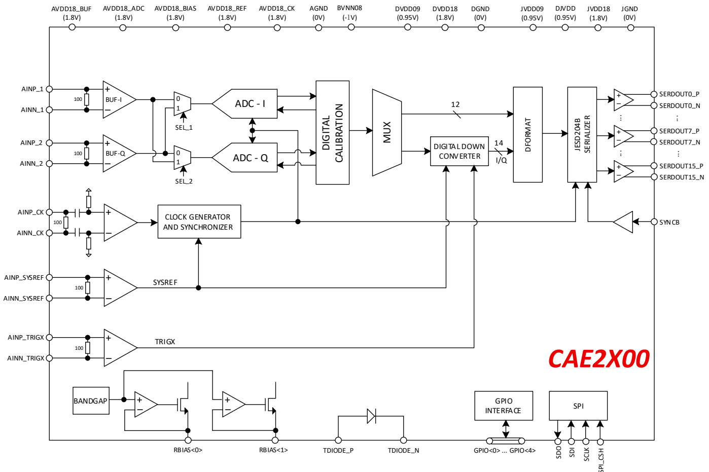
图 8-1. 功能框图
