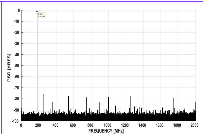
图 7-4. FFT at Fin = 180MHz, 4GSPS (0.8Vpp FS)
