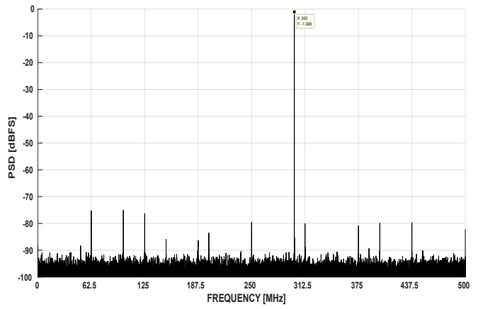
图 7-18. FFT at Fin = 300MHz, 1GSPS (1Vpp FS)
