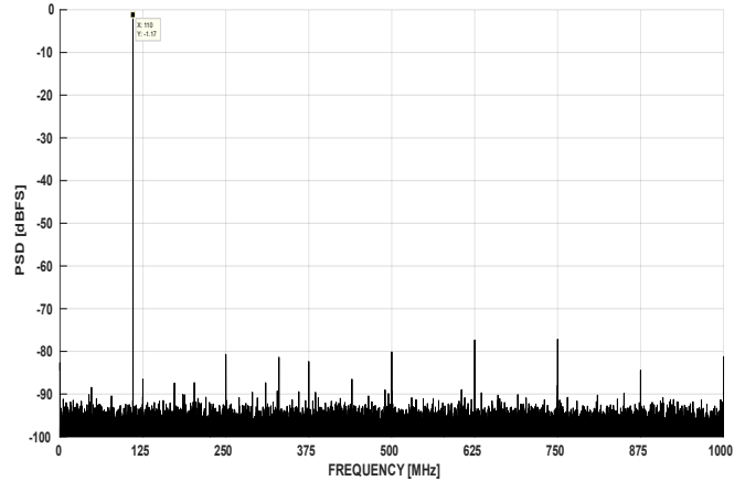
图 7-10. FFT at Fin = 110MHz, 2GSPS (1Vpp FS)
