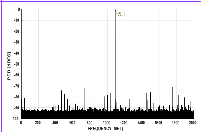
图 7-6. FFT at Fin = 1.09GHz, 4GSPS (0.8Vpp FS)
