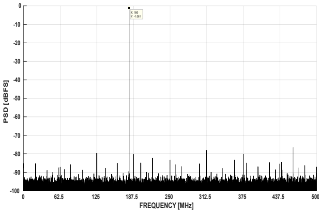
图 7-17. FFT at Fin = 180MHz, 1GSPS (1.0Vpp FS)
