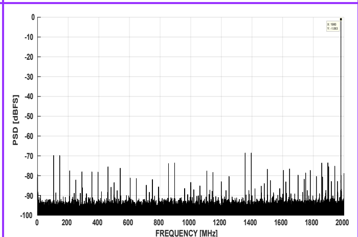
图 7-8. FFT at Fin = 1.98GHz, 4GSPS (1.0Vpp FS)
