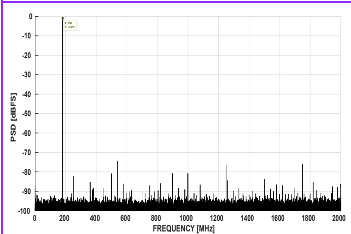
图 7-5. FFT at Fin = 180MHz, 4GSPS (1.0Vpp FS)
