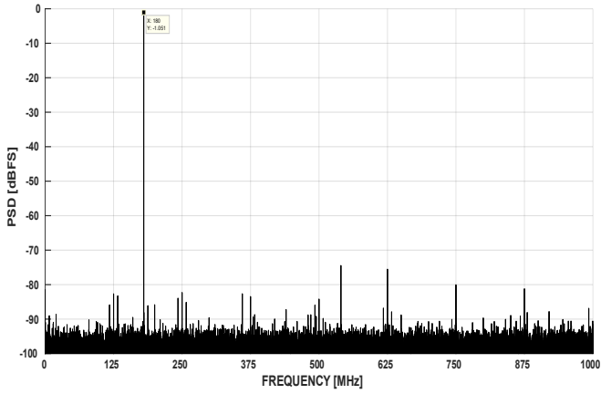
图 7-11. FFT at Fin = 180MHz, 2GSPS (1Vpp FS)
