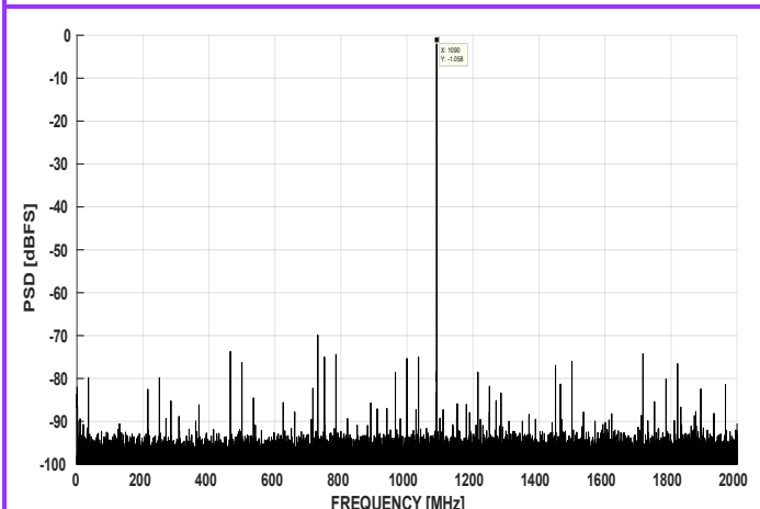
图 7-7. FFT at Fin = 1.09GHz, 4GSPS (1.0Vpp FS)
