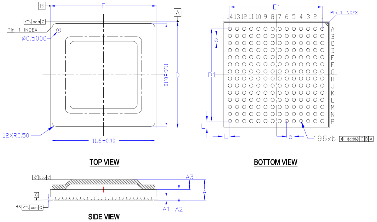
图 10-1. FCBGA196 封装尺寸图
